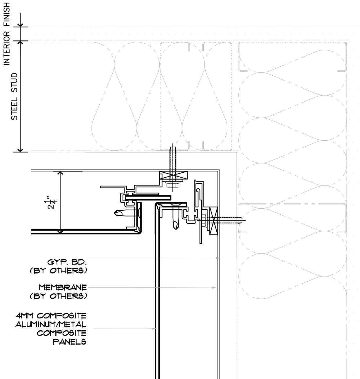
10 INSIDE CORNER RS SCALE: 6" = 1'-0"
